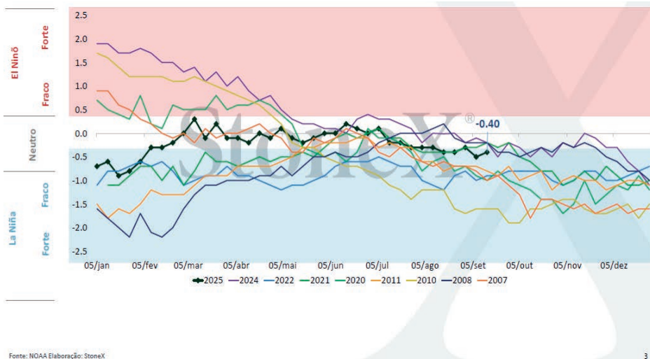
Gráfico 01 – Histórico da temperatura da água do oceano Pacífico.
